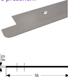
Spodní provedení s přesahem
