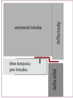
Umístění spodní ochranné lišty MT/spodniS (pohled z boku)
