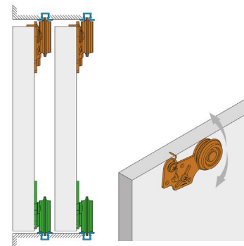
KOLEČKA S KULIČKOVÝM LOŽISKEM
