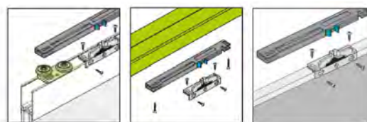
způsoby montáže tlumení
