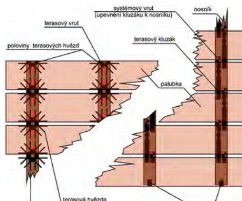
Schéma kladení terasových hvězd a kluzáků
