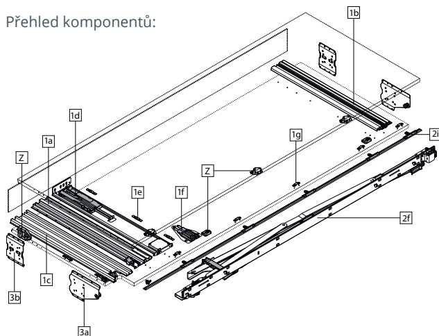
MONTÁŽ KAPSY
