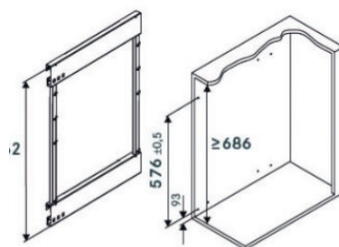
MONTÁŽNÍ NÁVOD
