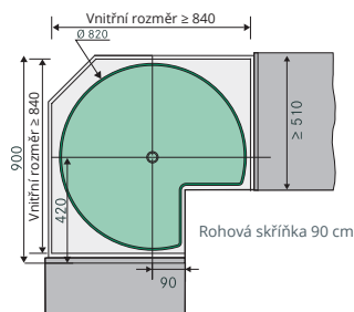
MONTÁŽNÍ NÁVOD
