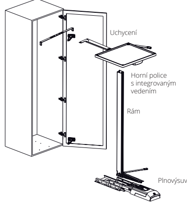
MONTÁŽNÍ NÁVOD
