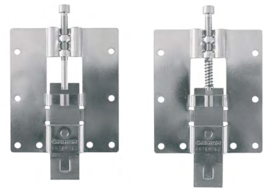
horní závěs
