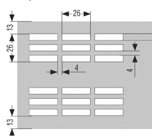
Výsek B2
