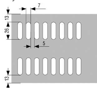
Výsek A2
