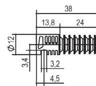
korpusový díl
