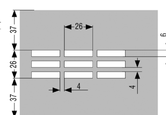
Výsek B1
