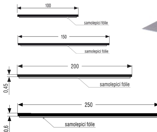
Výsek B2
