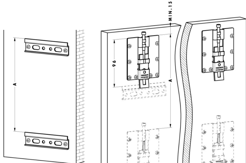
spodní závěs
