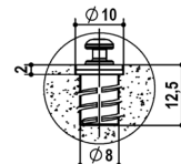
korpusový díl
